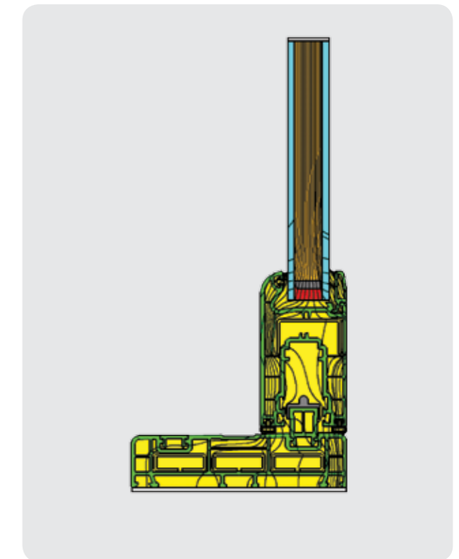
WINDOW HEAT FLOW DIAGRAM UF:1,7 W/M² °K UW: 1,6 W/M² °K
