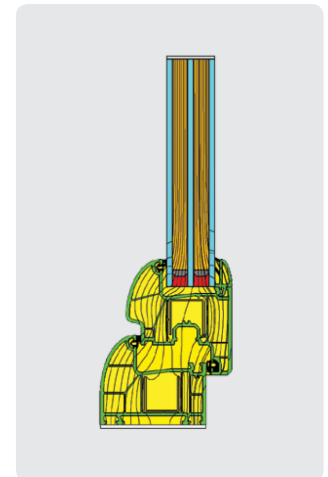
WINDOW HEAT FLOW DIAGRAM UF:1,1 W/M² °K UW: 1,15 W/M² °K
